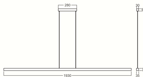
Pendente 4141 LED: 68,4W - 7600 lm - 3000 K ou 6000 K 127V ou 220V Luminária: 1930 x 35 x 35 mm Base de teto: 280 x 30 x 35 Cabos de alimentação: 2 m (reguláveis)
