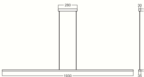
Pendente 4129 LED: 68,4W - 7600 lm - 3000 K - 127V ou 220V Luminária: 1930 x 35 x 20 mm • Luz indireta Base de teto: 280 x 30 x 35 Cabos de alimentação: 2 m (reguláveis)
