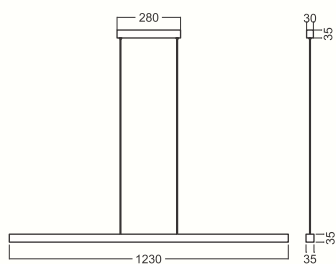
Pendente 4139 LED: 43,2W - 4800 lm - 3000 K ou 6000 K 127V ou 220V Luminária: 1230 x 35 x 35 mm Base de teto: 280 x 30 x 35 Cabos de alimentação: 2 m (reguláveis)
