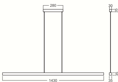
Pendente 4140 LED: 50,4W - 5600 lm - 3000 K ou 6000 K 127V ou 220V Luminária: 1430 x 35 x 35 mm Base de teto: 280 x 30 x 35 Cabos de alimentação: 2 m (reguláveis)
