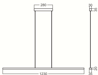
Pendente 4127 LED: 43,2W - 4800 lm - 3000 K - 127V ou 220V Luminária: 1230 x 35 x 20 mm • Luz indireta Base de teto: 280 x 30 x 35 Cabos de alimentação: 2 m (reguláveis)
