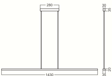
Pendente 4128 LED: 50,4W - 5600 lm - 3000 K - 127V ou 220V Luminária: 1430 x 35 x 20 mm • Luz indireta Base de teto: 280 x 30 x 35 Cabos de alimentação: 2 m (reguláveis)
