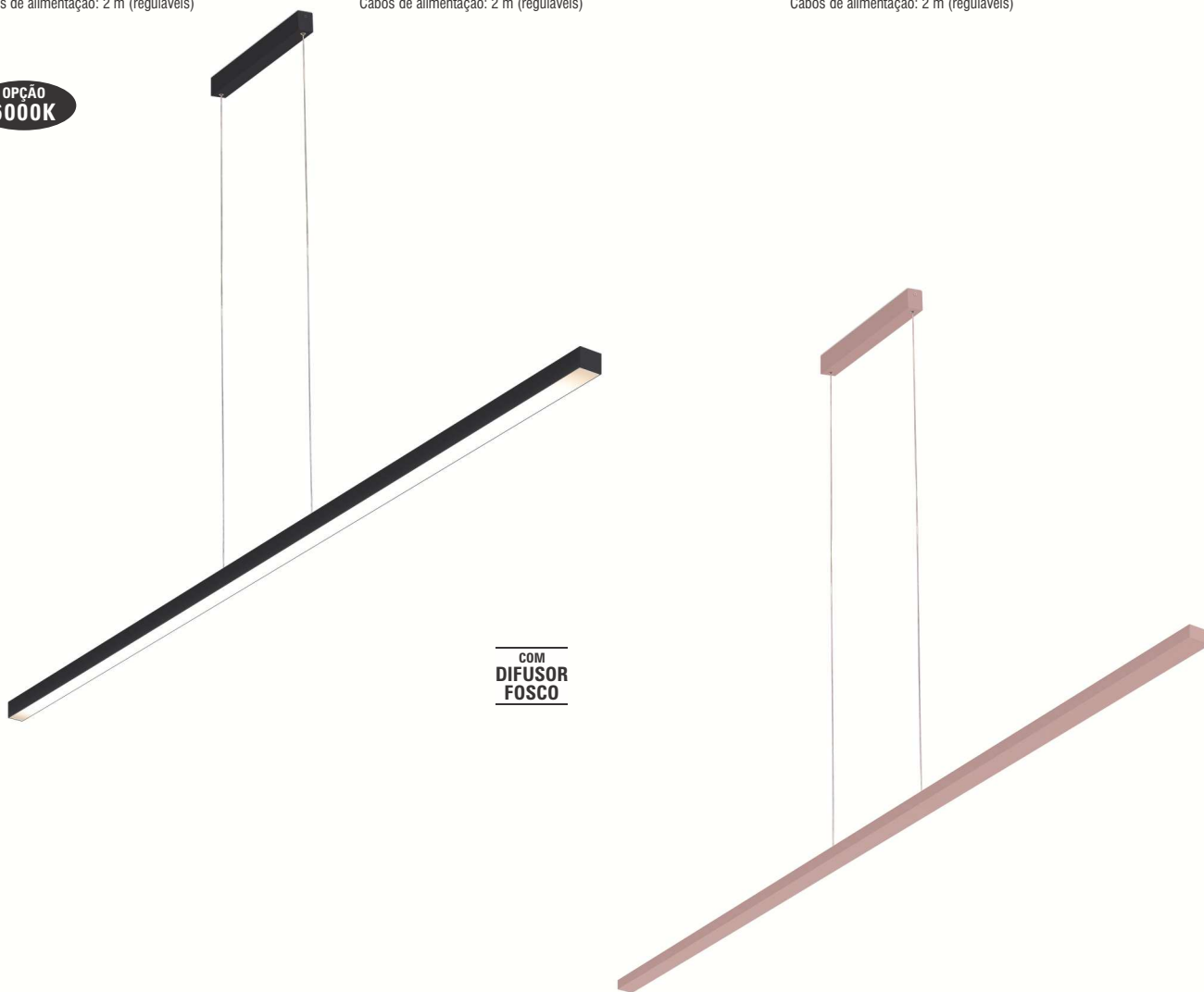
Pendente 4139 LED: 43,2W - 4800 lm - 3000 K ou 6000 K 127V ou 220V Luminária: 1230 x 35 x 35 mm Base de teto: 280 x 30 x 35 Cabos de alimentação: 2 m (reguláveis)
