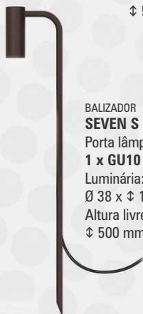
BALIZADOR SEVEN S 1321 Com base Porta lâmpada: 1 x GU10 MR11 Luminária: Ø 38 x ϕ 100 mm Base: Ø 100 x 2 mm Altura livre: ϕ 500 mm
