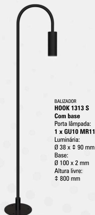
BALIZADOR HOOK 1312 S Porta lâmpada: 1 x GU10 MR11 Luminária: ∅ 38 x ∅ 90 mm Altura livre: ∅ 800 mm
