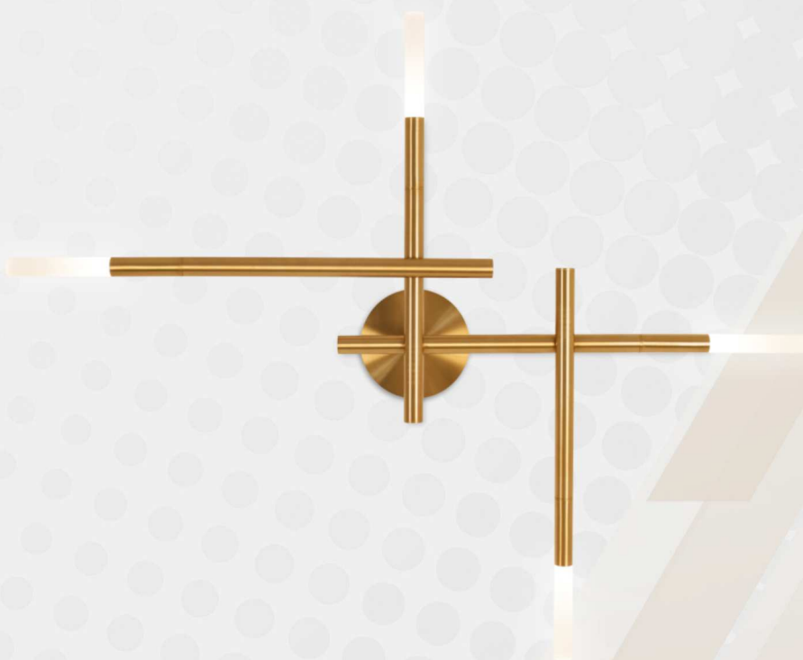
ARANDELA STEP 1691 Porta lâmpadas: 4 x G9 Halopin Difusor: Acrílico fosco Luminária total: ↔ 1040 x ⌀ 840 mm Base de parede: Ø 120 x 15 mm c/ blanquet de Ø 150 mm Profundidade: ↗ 120 mm
