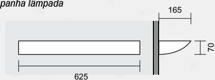
ARANDELA 4036 P Porta lâmpada: 1 x G13 T8 LED Tubular (T8 600 mm) Luminária: \Leftrightarrow 625 x \varnothing 70 mm Profundidade: \nearrow 165 mm * Não acompanha lâmpada
