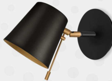
ARANDELA RAVENA POCO MOBILE 4059 Porta lâmpada: 1 x E27 Tamanho da cúpula: Ø 125 x ϕ 125 mm Luminária total: ⇔ 125 x ϕ 145 mm Base de parede: Ø 120 x 15 mm c/ blanquet de Ø 150 mm Profundidade: ⌈ 175 mm
